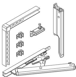
Comando vasistas
