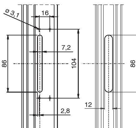
Cremone machining art. 01164N, 01165N
