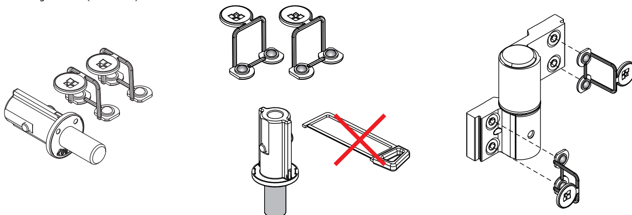
Código 05243 (kit 2 abas)
