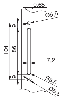
Usinagem do entre-eixos 104 mm versão monodirecional
