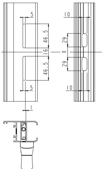
Usinagem tipo 1
