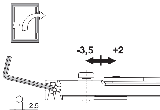
Regulagem da queda da folha
