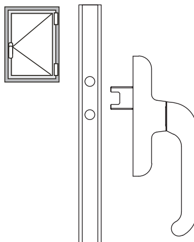
Usinagem do entre-eixo de 98 mm
