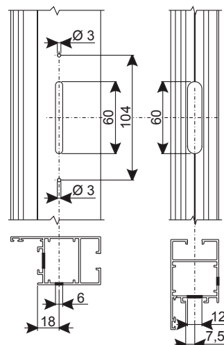
Usinagem para versões bidirecionais
