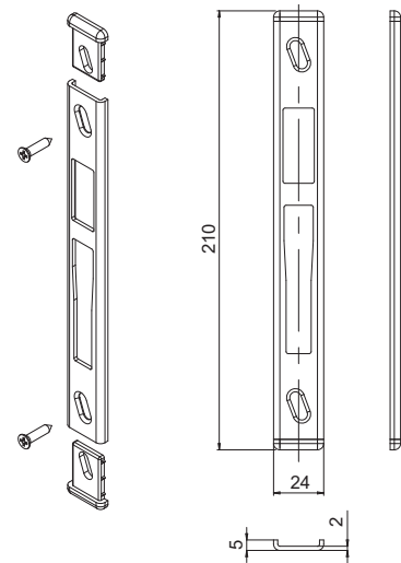
Contrafechos Tipo 6
