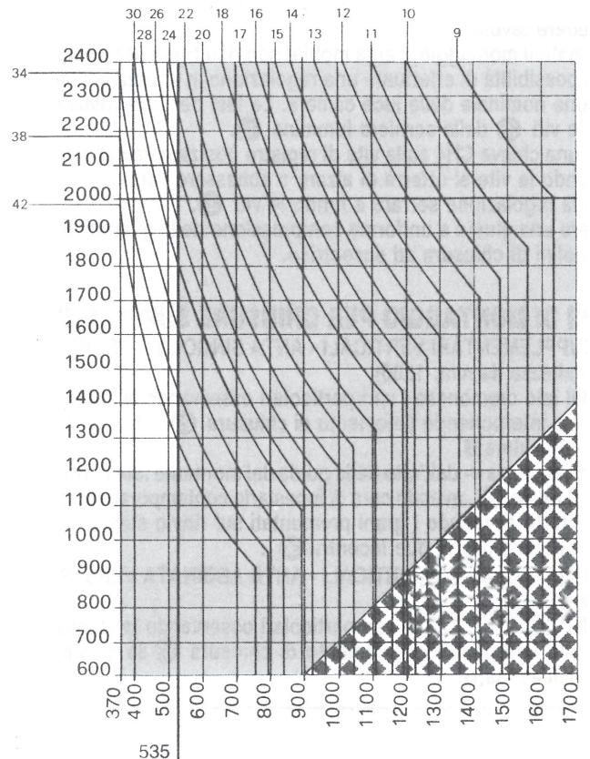
Gráfico de dimensões e capacidade de carga para cód.: 04516, 04518
