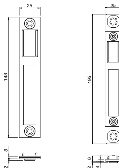
Tipo 2 – cód. 07695
