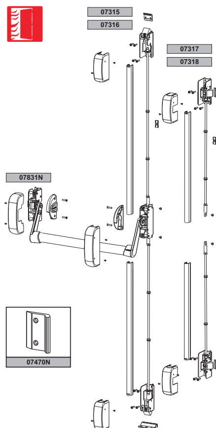
Versão corta fogo
