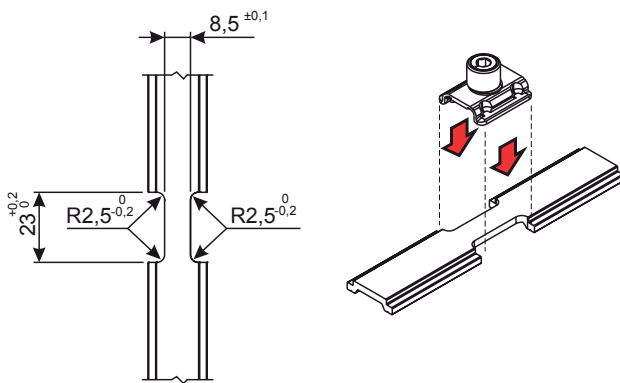
Usinagem da haste
