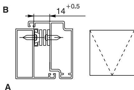
Maxim-ar (A: interno; B: externo)
