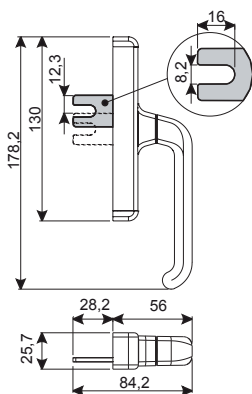
Usinagem do entre-eixos 108 mm versão bidirecional
