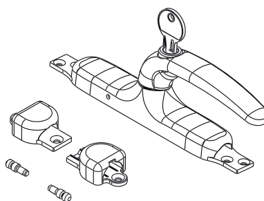
Cremona Provence com fecho a leva com chave
