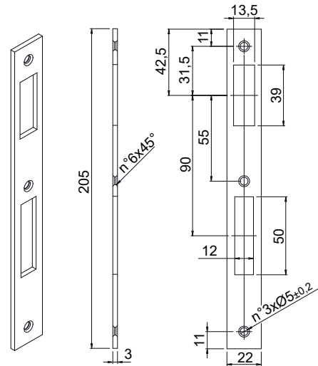
Controplaca Tipo 9
