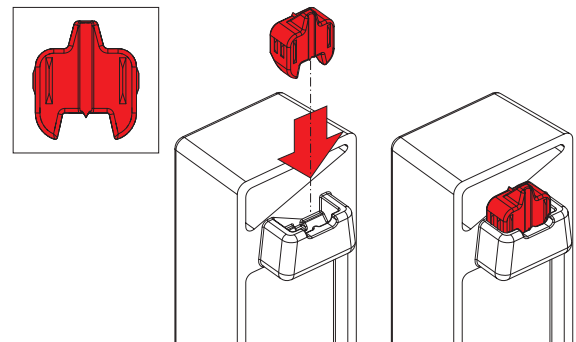
Art. 06014: bloqueio com 1 dente
