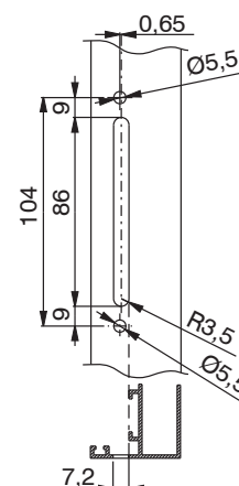
Usinagem do entre-eixo de 104 mm
