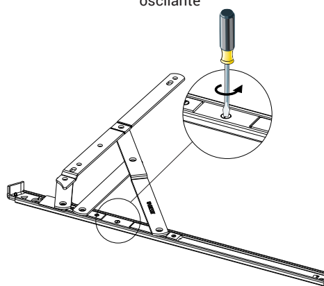
Elemento de desbloqueio para a limpeza do lado externo do oscilante
