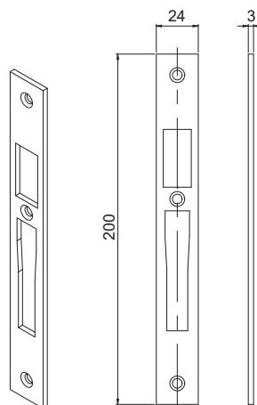
Contrafechos Tipo 3
