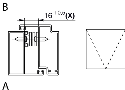
Maxim-ar (A: interno; B: externo)
