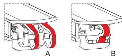
A: mola de 2 dentes - B: mola de 1 dente
