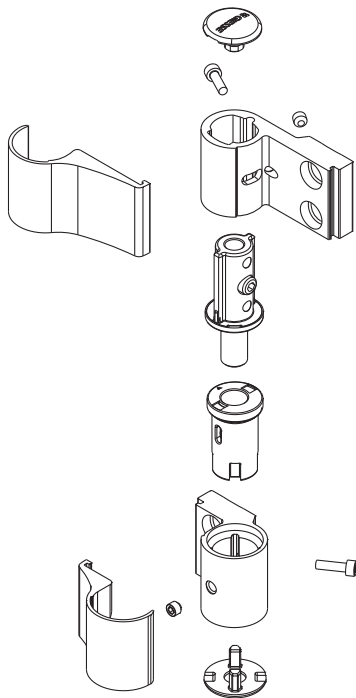
Regulagem em altura
