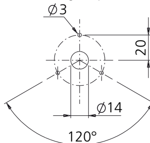
Usinagem tipo 2
