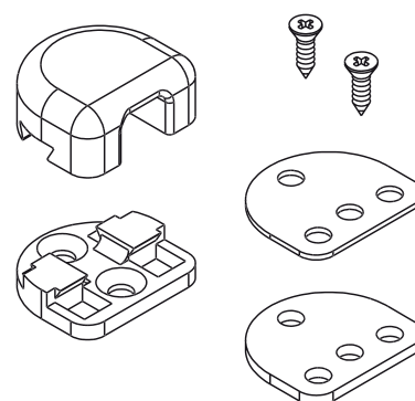
Encontro de abertura externa
