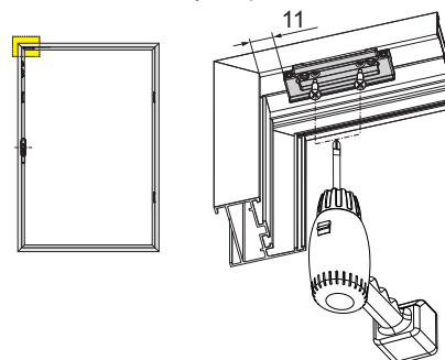
Calço superior
