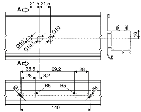
Tipo C: usinagens
