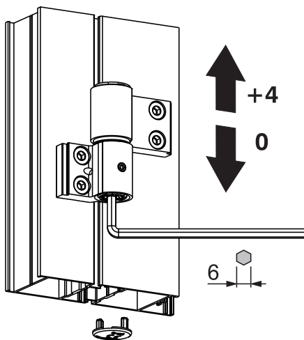
Regulagem em altura
