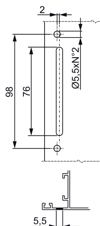
Usinagem do entre-eixo de 98 mm
