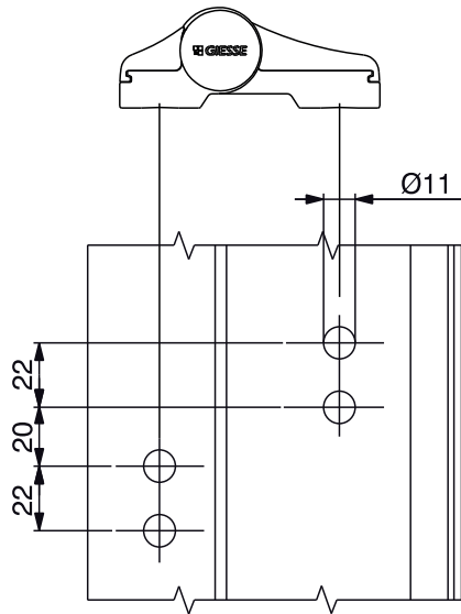
Usinagem no perfil (2 abas)
