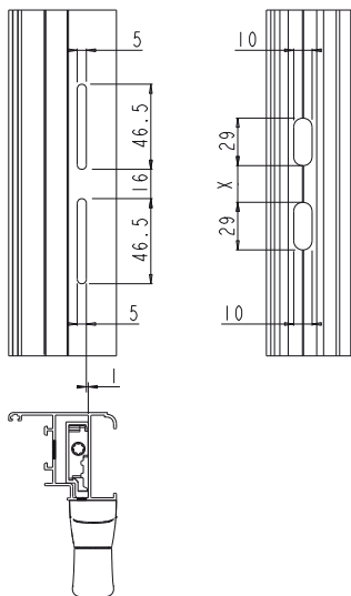
Usinagem tipo 2
