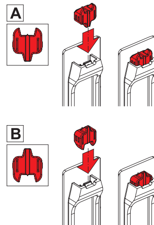
Preparação da maçaneta - A: 2 dentes - B 1 dente
