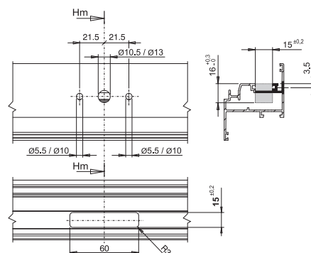
Tipo C: usinagens
