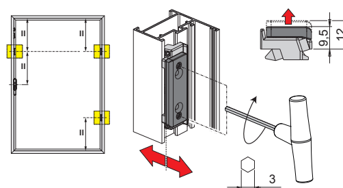
Calço superior
