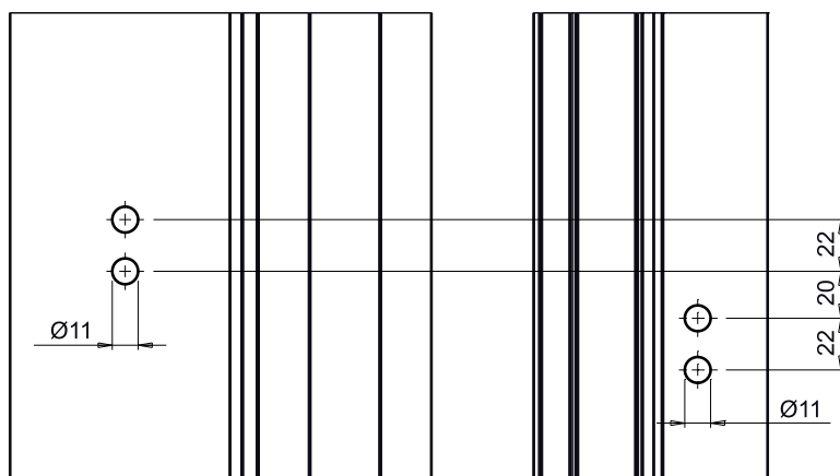
Usinagens no perfil
