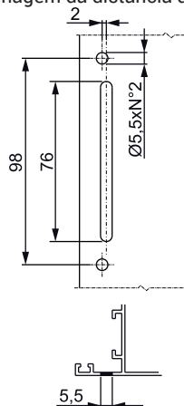
Usinagem da distância de 98
