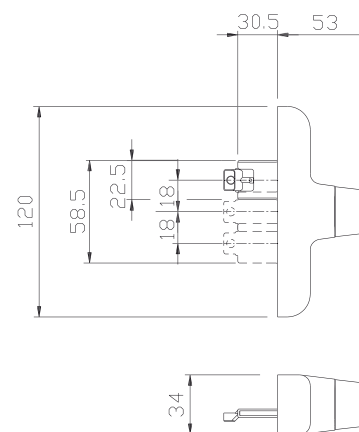
Versão abre e tomba
