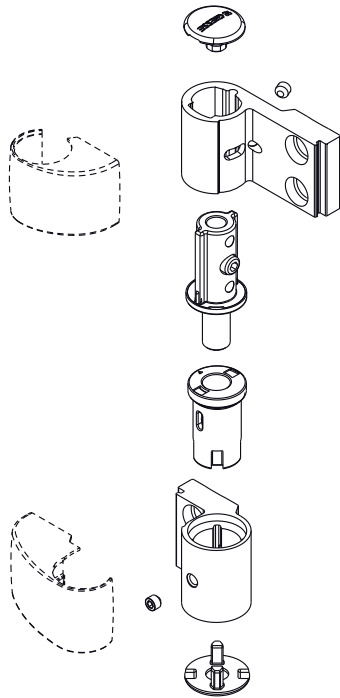
Regulagem em altura
