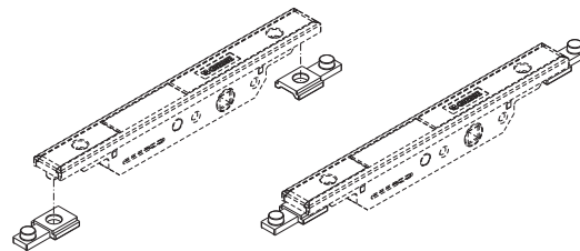
Montagem com movimento 0102001
