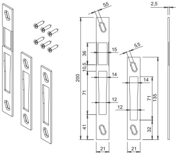
Contrafechos Tipo 5
