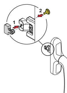
D3 - Montagem de calços para anti falsa mecanismo
