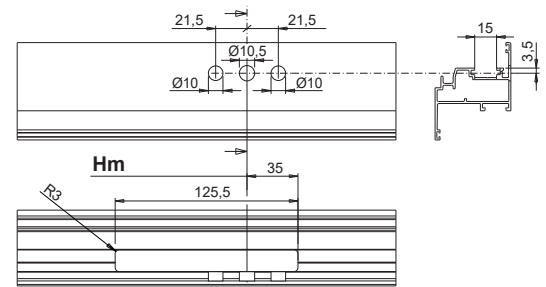
Tipo D: usinagens
