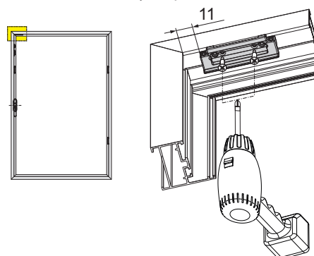
Calço superior
