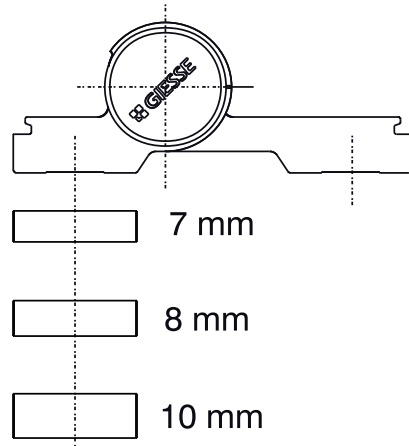
Grades sem casquilho
