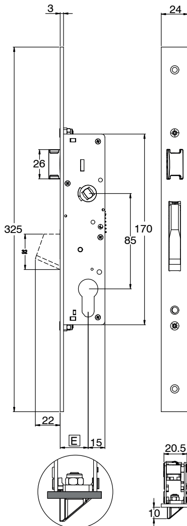
Frontal plano
