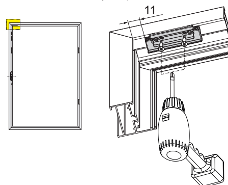
Calço superior
