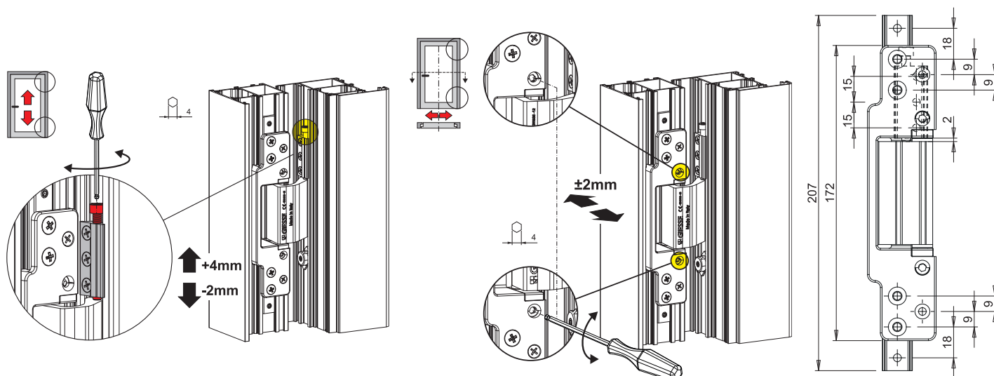
Regulagem em altura
