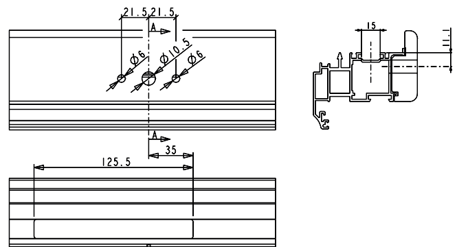
Tipo B: usinagens
