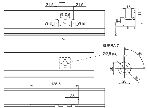
Tipo A: usinagens
