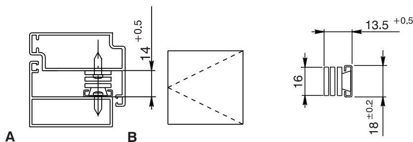
GIRO EXTERNO (A: interno; B: externo)
