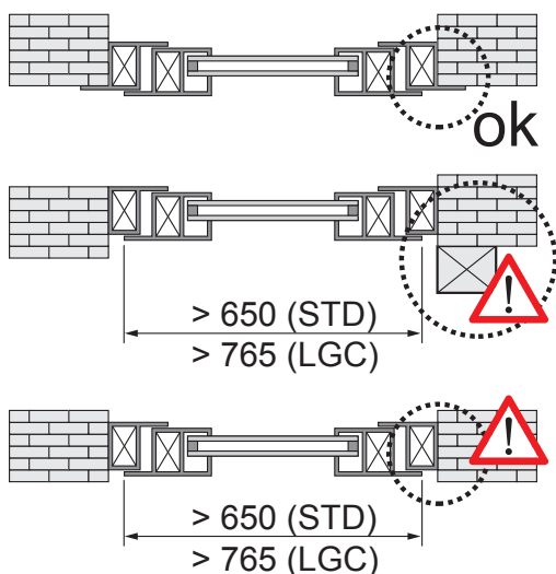
Obrigatória utilização do braço FRIZ
