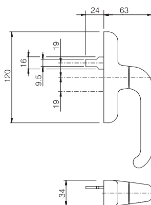
B. Versão monodirecional
