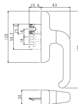
C. Versão monodirecional
