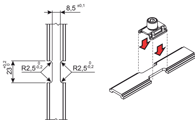
Lavorazione astina
