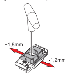
Regolazione compressione
