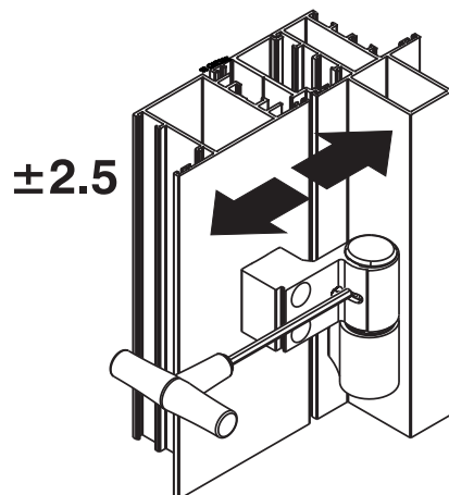
Regolazione laterale
