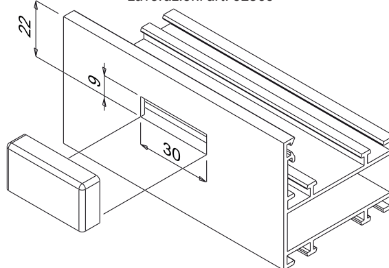
Lavorazioni art. 03195
