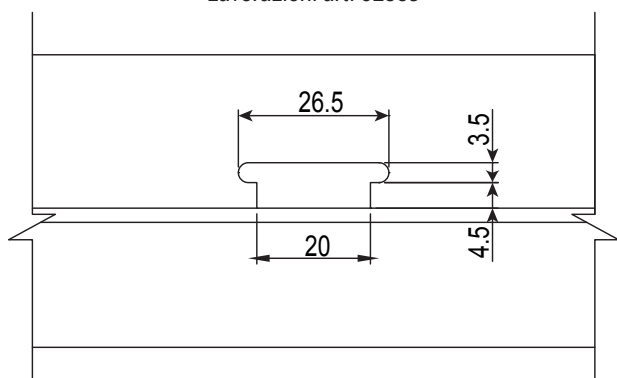
Lavorazioni art. 02359
