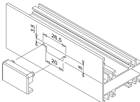
Lavorazioni art. 02328
