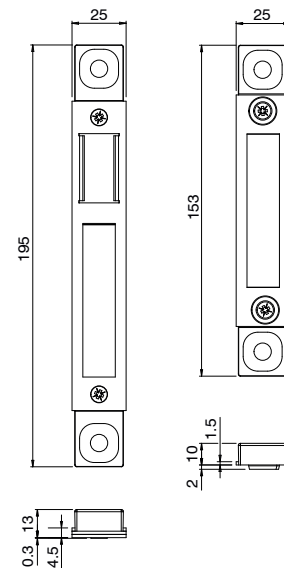
Tipo 5 – art. 07704
