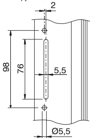
подготовка профиля под установку ручки С/С 98 мм
