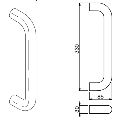
Ручка скоба "ПРЯМАЯ" из латуни
