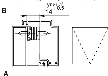
Верхняя подвеска (А: помещение, В: улица)
