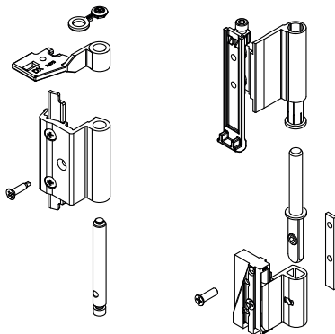
Обязательное использование штанги FRIZ
