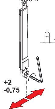
Регулирование шпингалета с артикулом 04347
