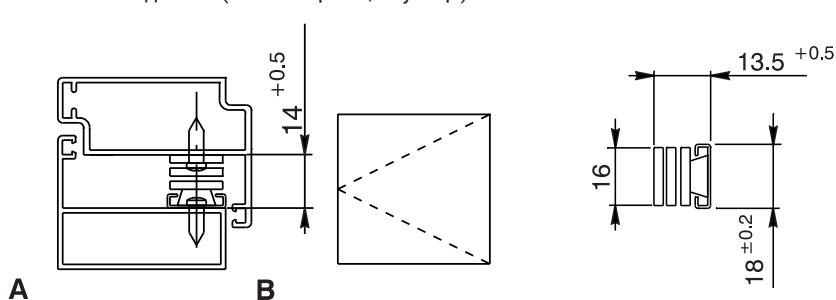
Боковая подвеска (А: помещение, В: улица)
