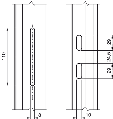
подготовка профиля под установку ручки арт. 01154001, 01155001
