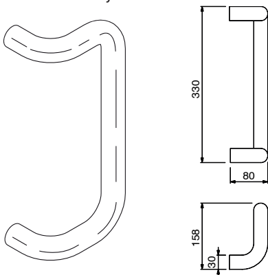
Ручка скоба "ИЗОГНУТАЯ" из латуни
