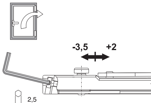
Регулировка верхнего перекоса
