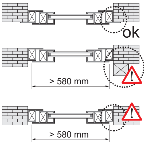
Обязательное использование штанги FRIZ
