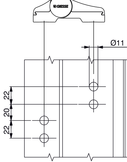
Подготовка профиля под петлю в двух секциях
