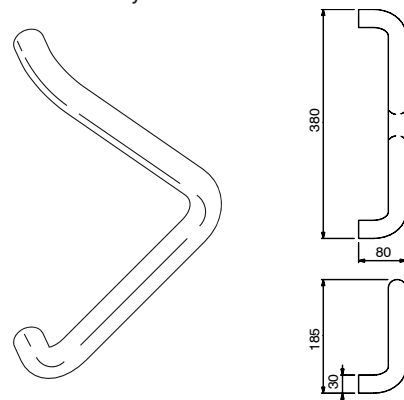
Ручка скоба "УГОЛ" из латуни
